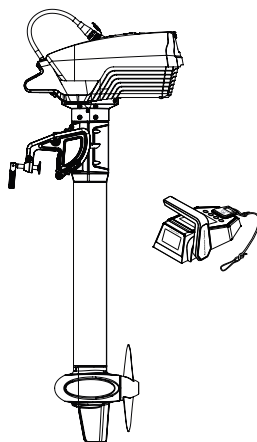
Spirit 1.0 Evo mit Spirit Batterie PLUS/Evo und Evo Fernsteuerung Kurzschaft 62,5 cm, 05571 Langschaft 75 cm, 05573
